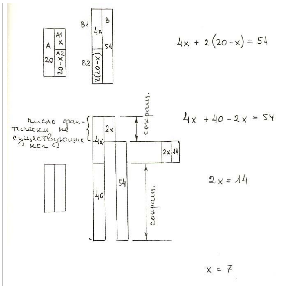
.262. Фиг.31. Алгебраическое решение
