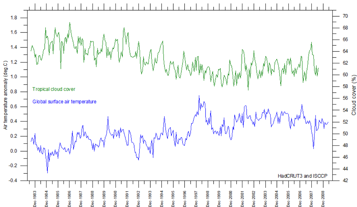
Рис. 5. Тропическое облачное покрытие ( 15^{\circ}\text{N} - 15^{\circ}\text{S} ) и глобальная среднемесячная поверхностная температура.
